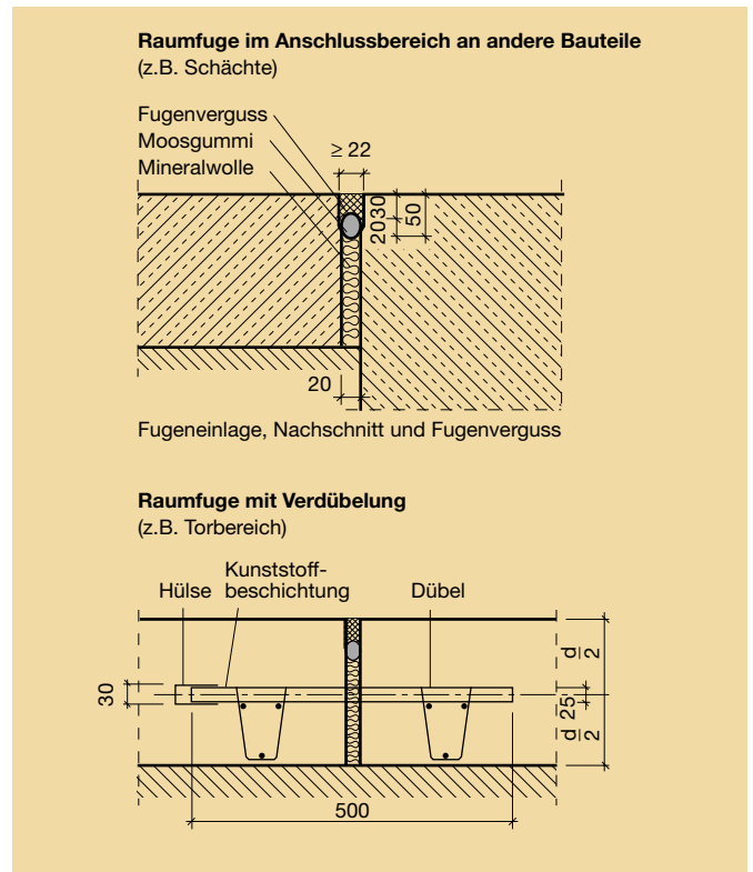
Bild 5: Bewegungsfugen mit Fugeneinlage mit und ohne Verdübelung [4]
